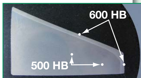
Geschliffene und geätzte Probe. In Epoxidharz eingebettet. Vorbereitet zur Metallographie.
