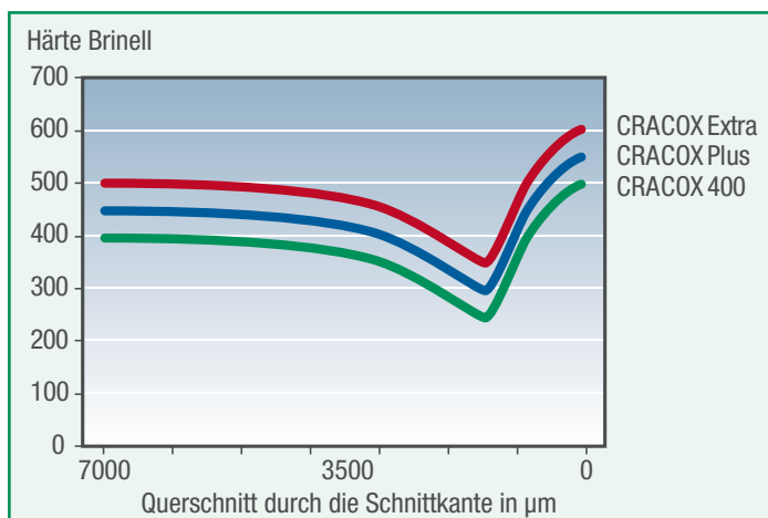
Aus unserem CRACOX Extra mit einer Ausgangshärte von ca. 500 HB wird an der Schnittkante ein 600 HB-Stahl!
